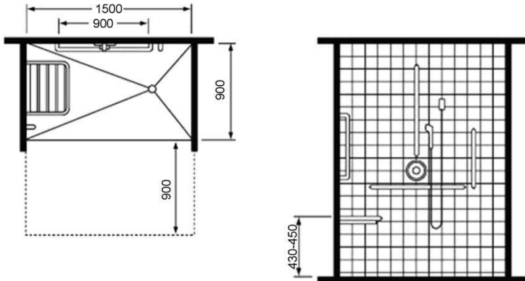
Рисунок 44 – Обладнання душової kabini
