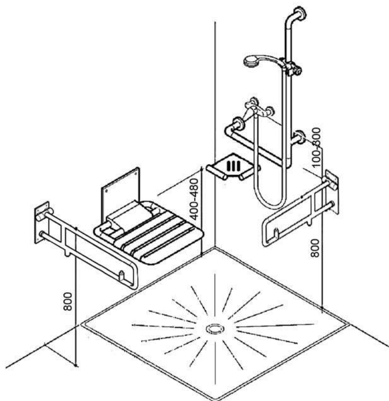
Рисунок 45 – Душова kabina з відкидним сидінням
