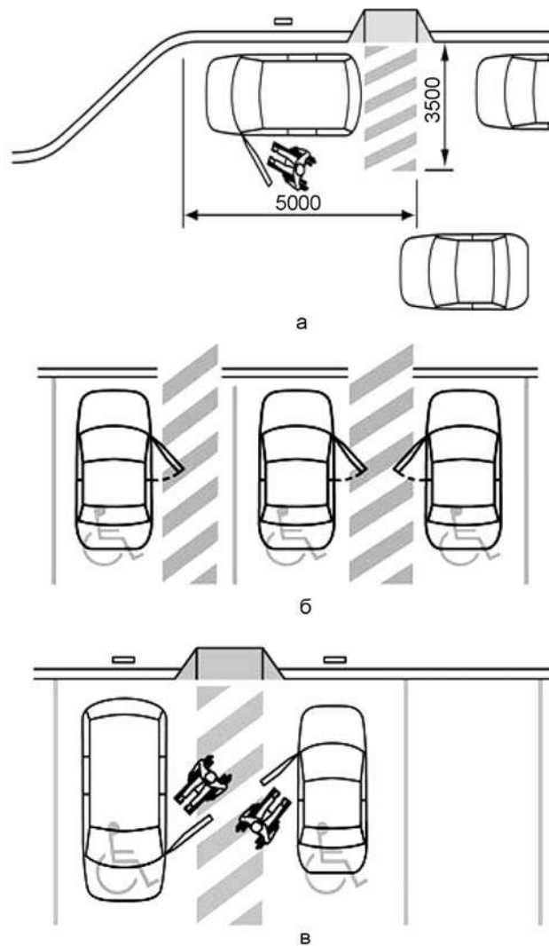
Рисунок 6 – Стоянки індивідуального транспорту для осіб з інвалідністю:
